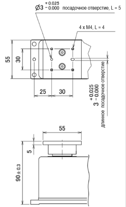
Вид с установленной дополнительной платформой (опция)
