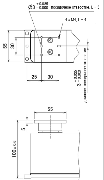
Вид с установленной дополнительной платформой (опция)
